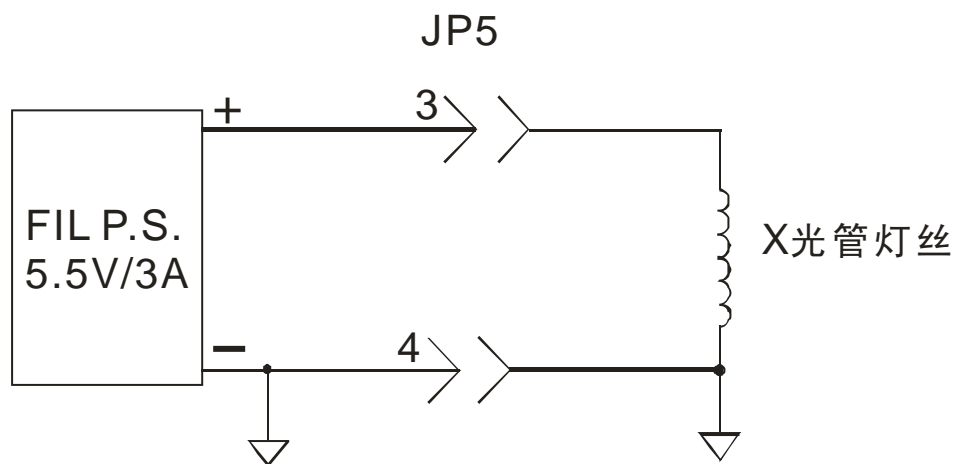
灯丝接线
