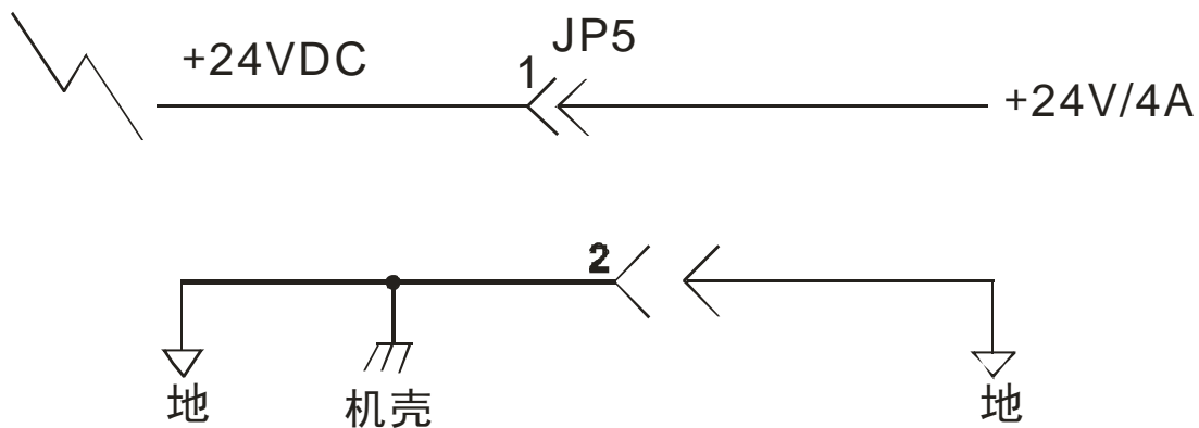
24V输入接线
