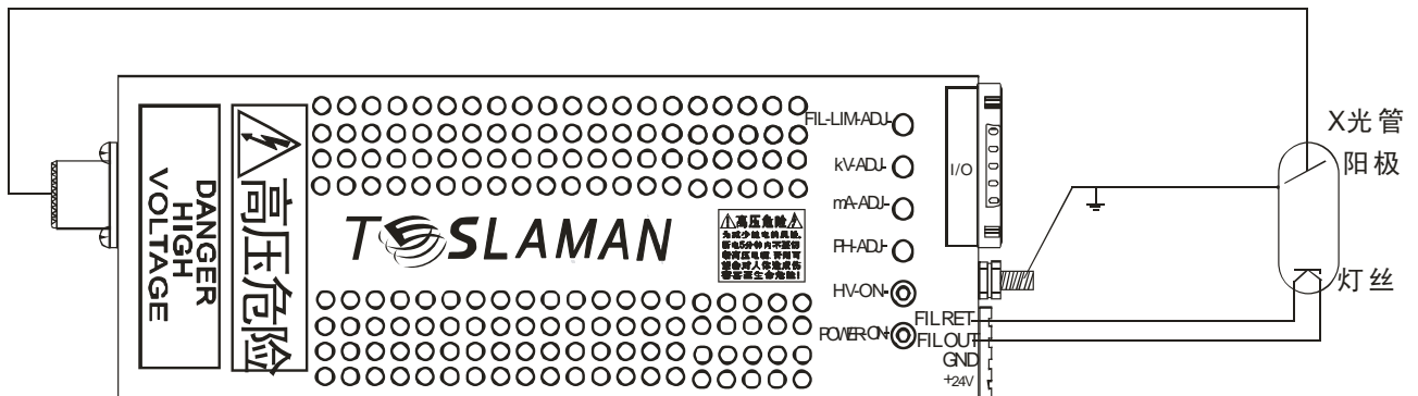
图 3.1 工作接线图
