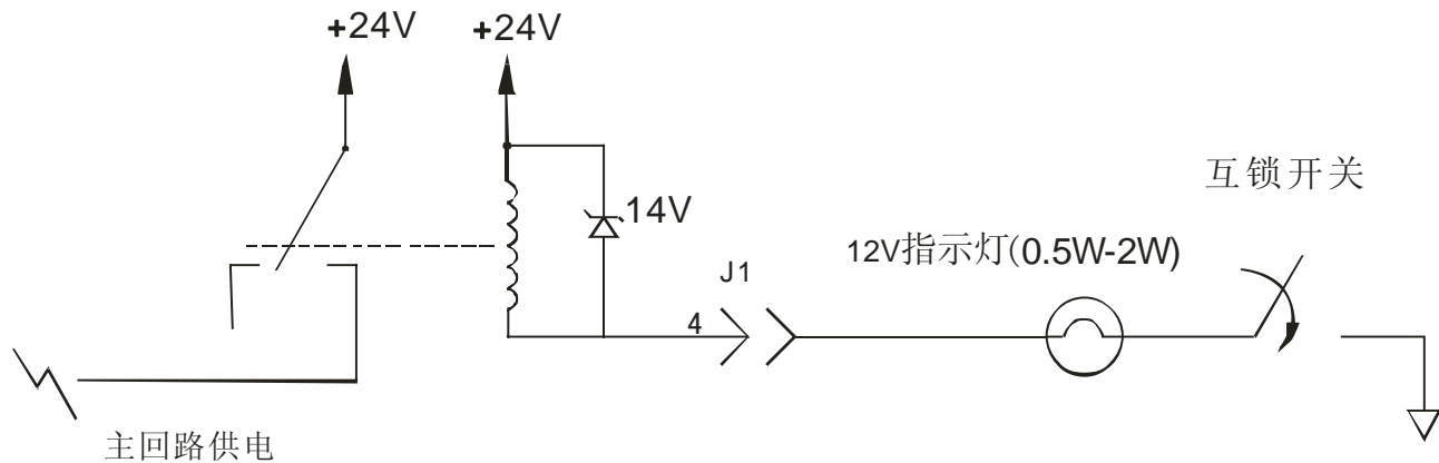
图 3.3 外部互锁接口
