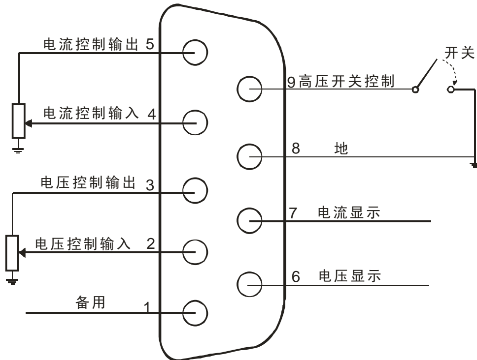
图 3.1 远程控制接线示意图
