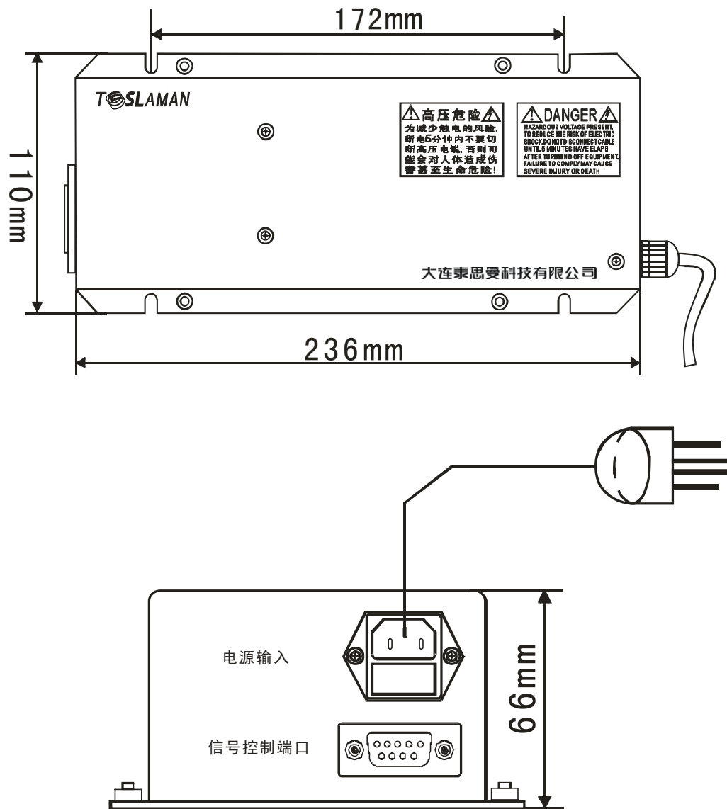
图 2.1 TAP4055 机械尺寸图
