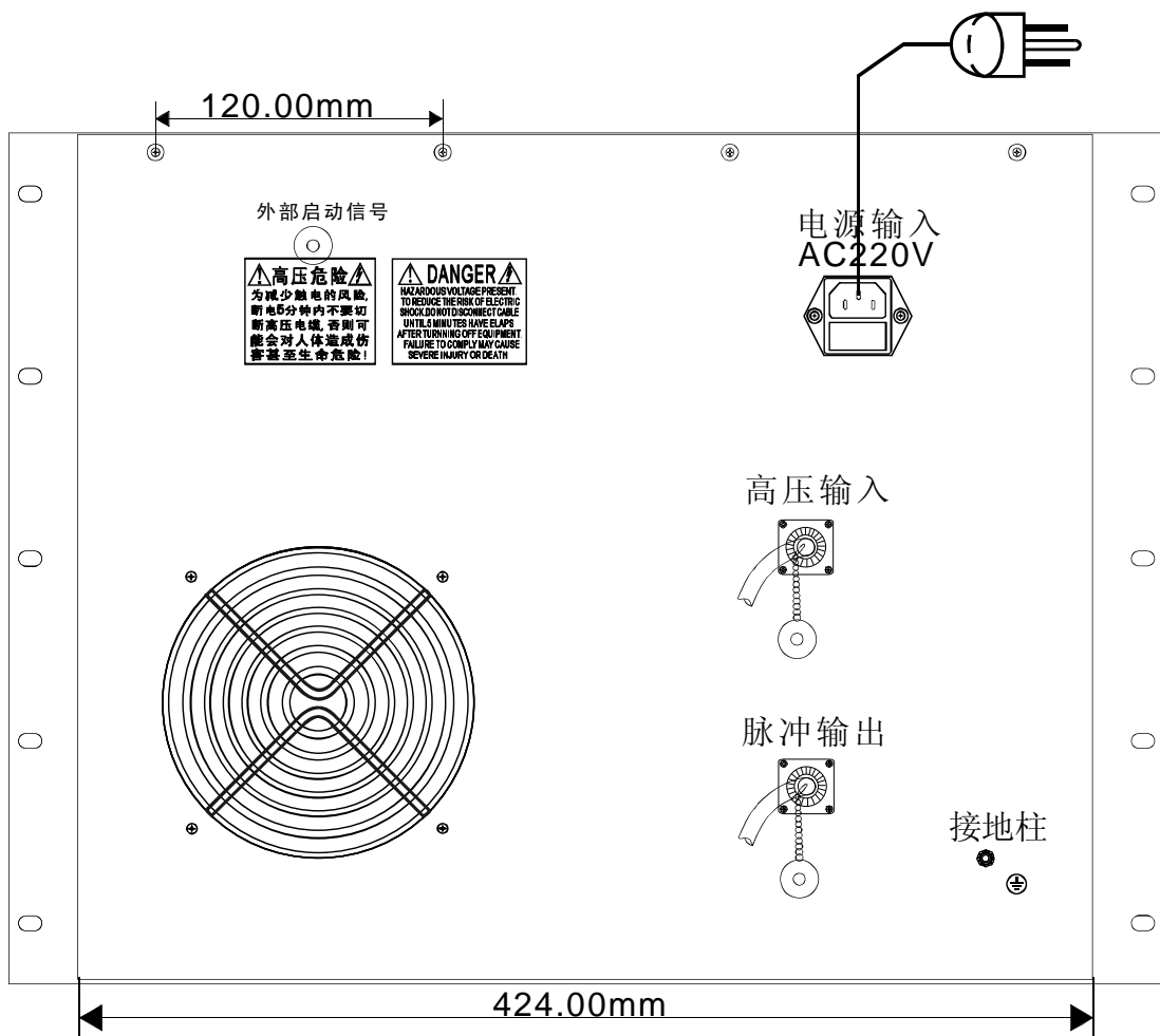
脉冲电源后面板
