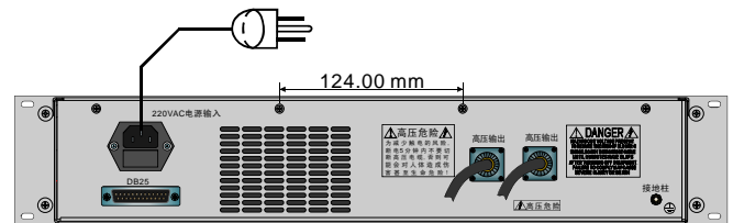
后端板
