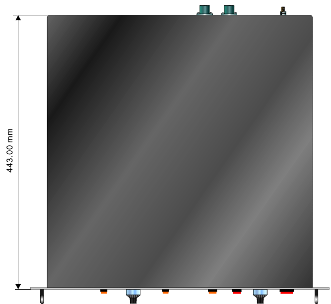
上盖板
